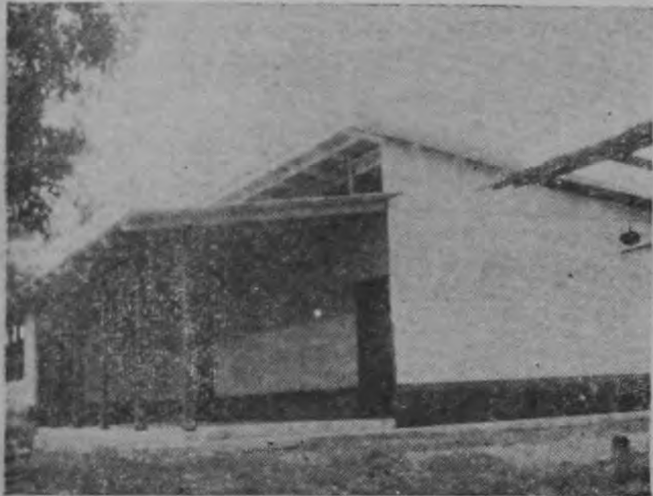
EL MOP CONSTRUYE ESCUELAS. — Este edificio escolar fue construido por el Ministerio de Obras Públicas, en su afán por ayudar a la educación del país, en Cerbatana de Puriscal. Consta de 4 aulas con capacidad para 160 alumnos, dirección, servicios sanitarios y amplios corredores para que jueguen los niños.
